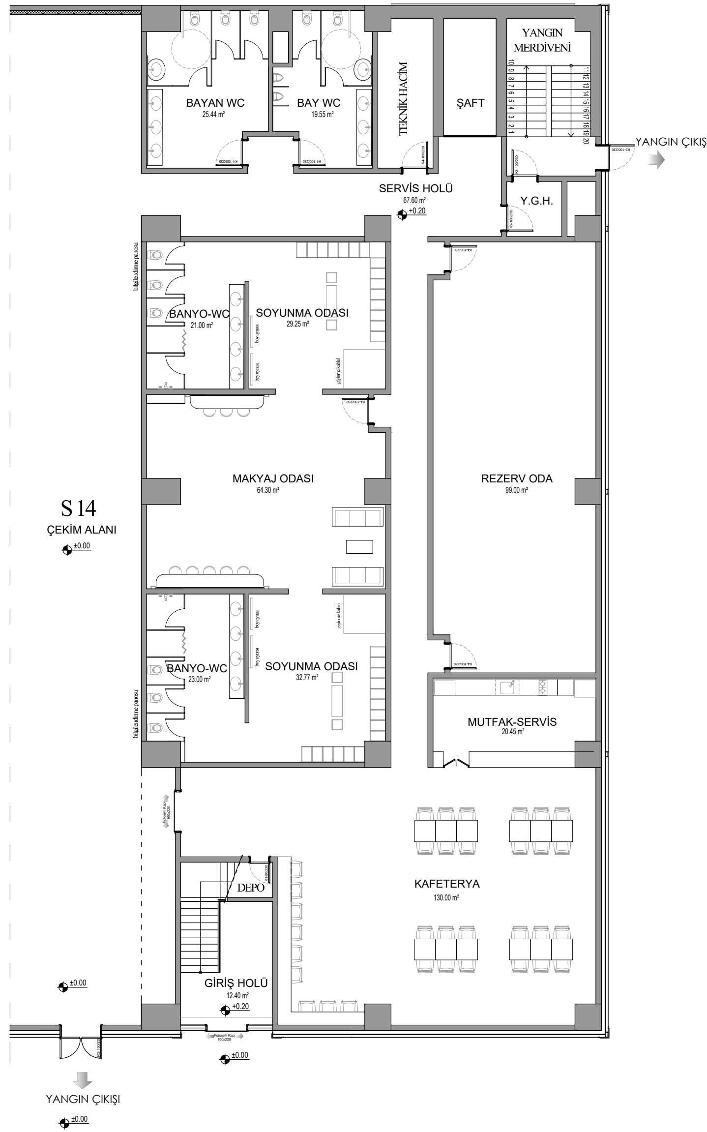
ZEMİN KAT PLANI
